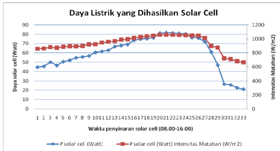
Gambar 11. Daya listrik solar cell
