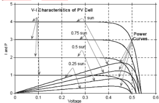
Gambar 4. Kurva karakteristik i-v terhadap perubahan iradiasi
