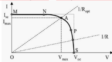
Gambar 2. Karakteristik kurva I-V solar cell
