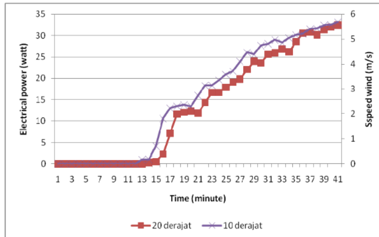
Gambar 12. Daya listrik turbin angin darrieus NACA airfoil 4 blade dengan sudut pitch 10^0 dan 20^0
