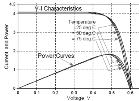
Gambar 3. Kurva karakteristik i-v terhadap perubahan temperatur
