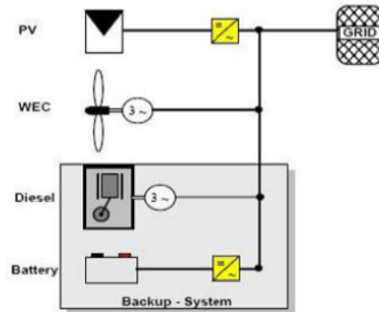
Gambar 7. Model pembangkit listrik hibrid
