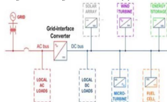
Gambar 2 Konsep arsitektur jaringan mikro
