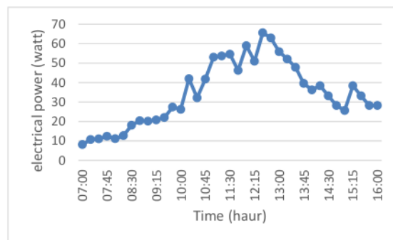
Gambar 5. Produksi listrik solar PV
