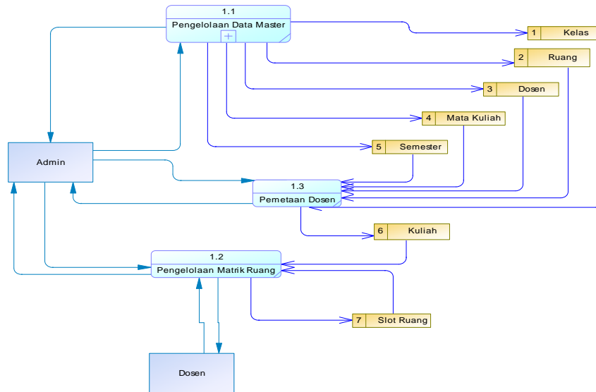
Gambar 3. DFD Reservasi Ruang Level 1
