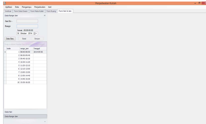
Gambar 10. Data Waktu
