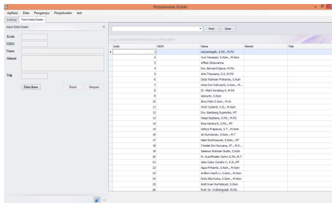
Gambar 8. Data Dosen
