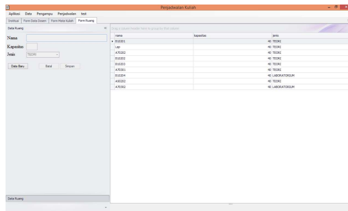
Gambar 11. Data Ruang
